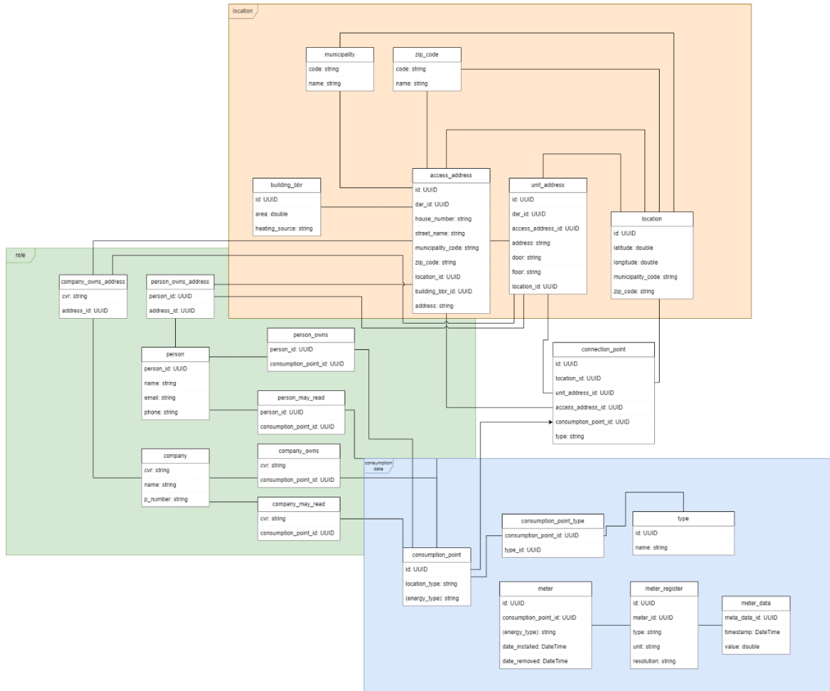
Figur 7 - Generisk Datamodel for Fjernvarmesektoren (Logisk)
